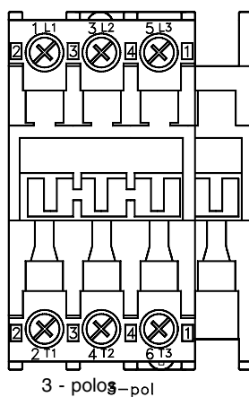
Marcado de bornes de contactor
