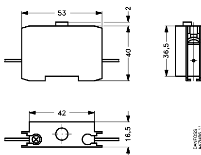
Temporizador electrónico con clip, ETB
