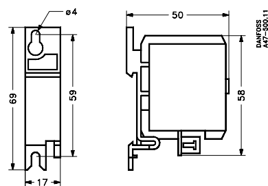
Acoplamiento RC para contactores CI 6, 9, 12, 15, 16, 20, 25, 30
