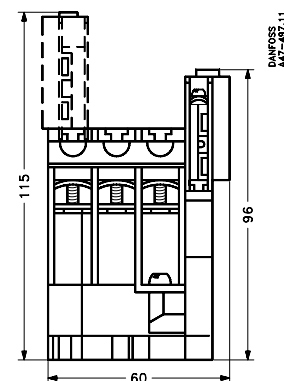
Montaje separado del módulo interface IFB
