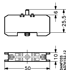
Montaje separado del temporizador electrónico con clip, ETB
