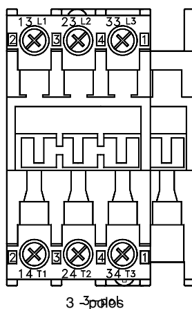
Marcado de bornes de relé
