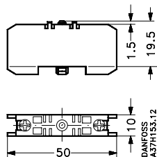
Bloque de contactos auxiliares CB
